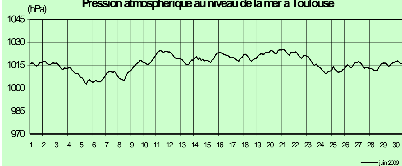
Pression atmosphérique au niveau de la mer à Toulouse
